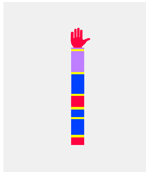
Julie Accentpaal met slagboom Hoogte: 2950mm Diameter: 323mm Lengte slagboom: 3800mm
